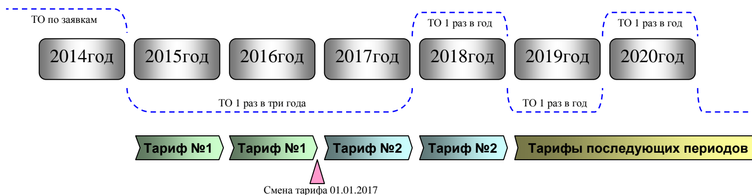
Схема выполнения работ по ТО ВКГО/ВДГО
